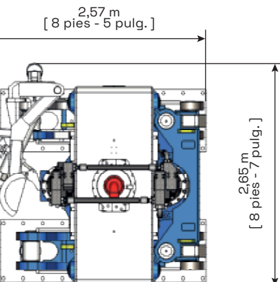
Máquina Retraído
