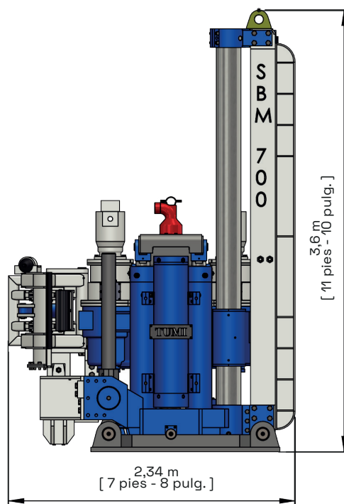
Máquina Retraído
